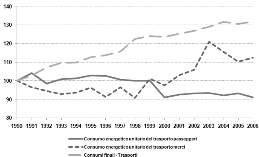
Fig. 11 Evoluzione consumi energetici finali e unitari nel settore dei trasporti in Italia
